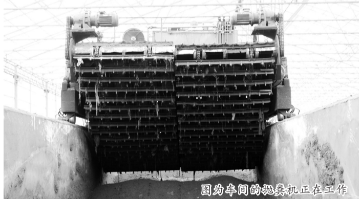
图为车间的抛粪机正在工作
